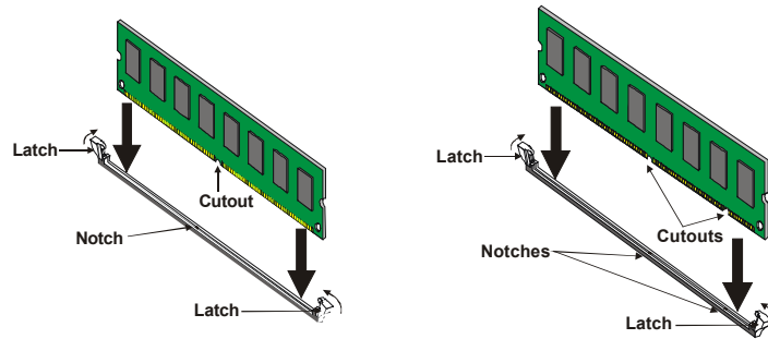
DDR SDRAM Module
